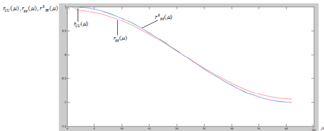
Рис.2 Графики нормированных корреляционных функций зашумленного сигнала r_{gg}(\mu) и полезного сигнала r_{UU}(\mu) , а также робастной корреляционной функции зашумленного сигнала r_{gg}^R(\mu) .
