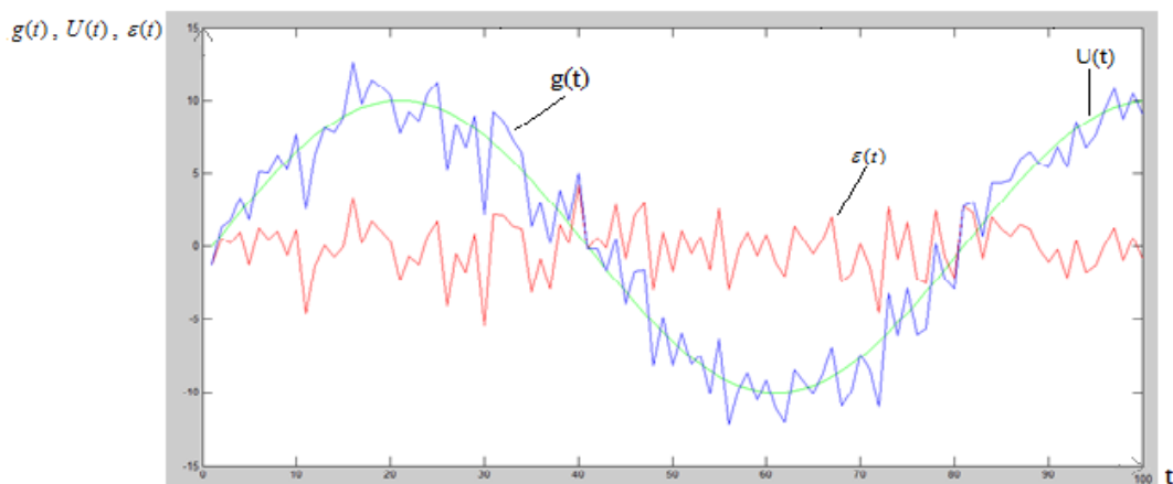
Рис.1 Графики изменения U(i\Delta t) , g(i\Delta t) и \varepsilon(i\Delta t) во времени
