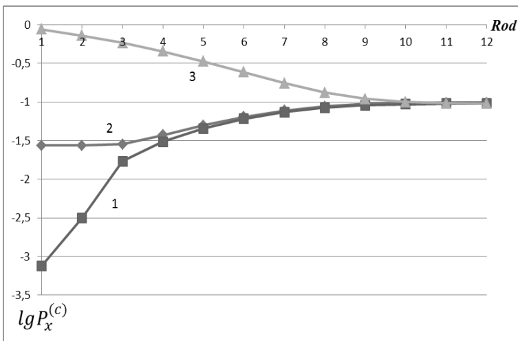
Şəkil 2. Kanalların bölünməsinin IPwCZv2-sxemindən istifadə zamanı müxtəlif tipli sorğuların itməsi ehtimallarının R_{od} parametrindən asılılığı, 1 – 1 - \lg P_{hv}^{(c)} ( \lg P_{hd}^{(c)} ), 2 – 1 - \lg P_{ov}^{(c)} , 3 – 1 - \lg P_{od}^{(c)} .
