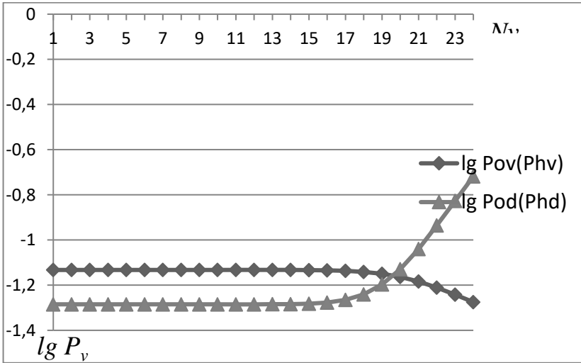
Şəkil 3. Kanalların bölünməsinin VPwCZv1-sxemi üçün danışıq sorğularının itməsi ehtimalının N_v parametrindən asılılığı
